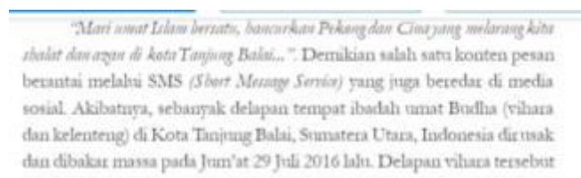
Gambar 4. berita provokatif
